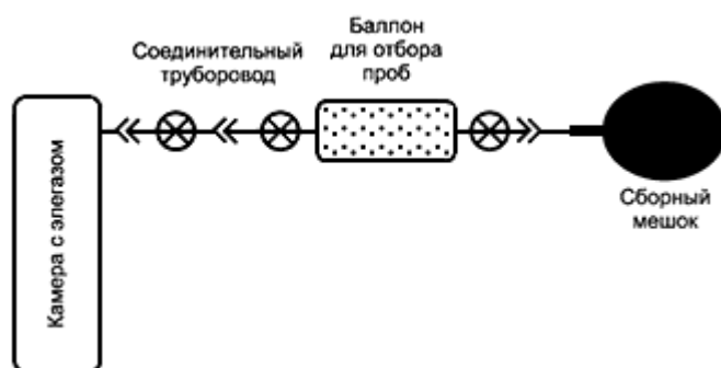
Рисунок В.2 - Установка для отбора газовой фазы элегаза: продувка
